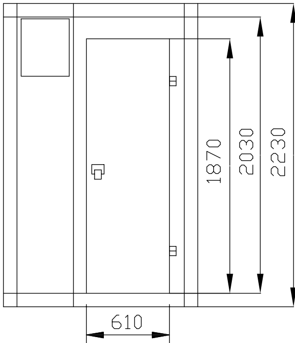
Zij aanzicht
